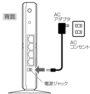
無線コンバータ LAN-HGW300/CV
